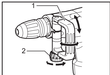
► 1. Poignée étrier latérale 2. Écrou de serrage
